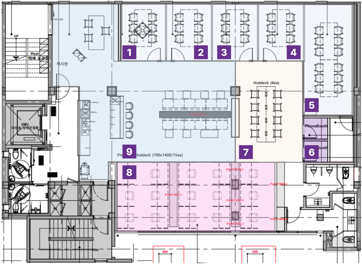
L층 배치도
